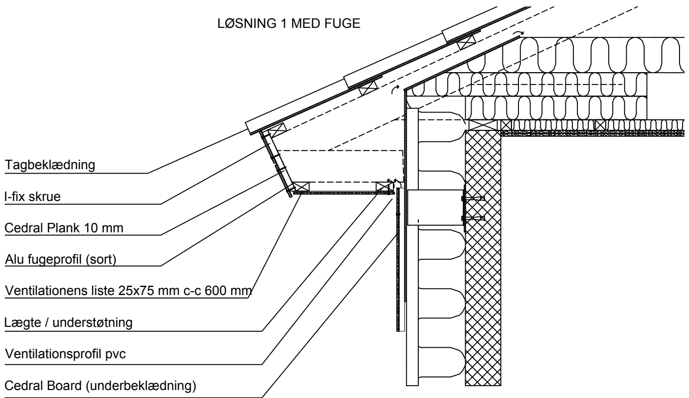
LODRET SNIT Fasade / udhæng
