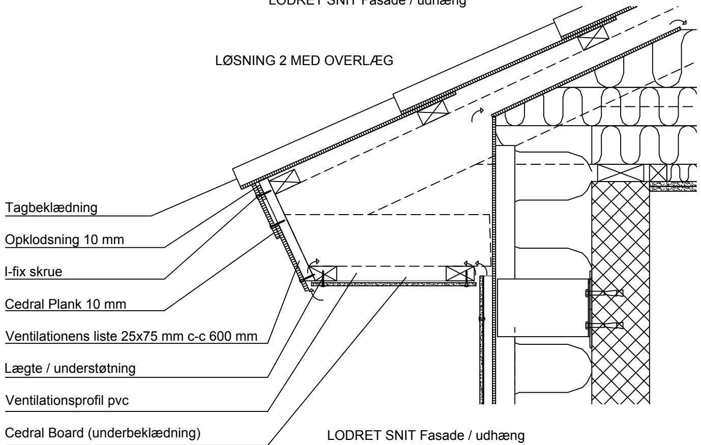
LODRET SNIT Fasade / udhæng
