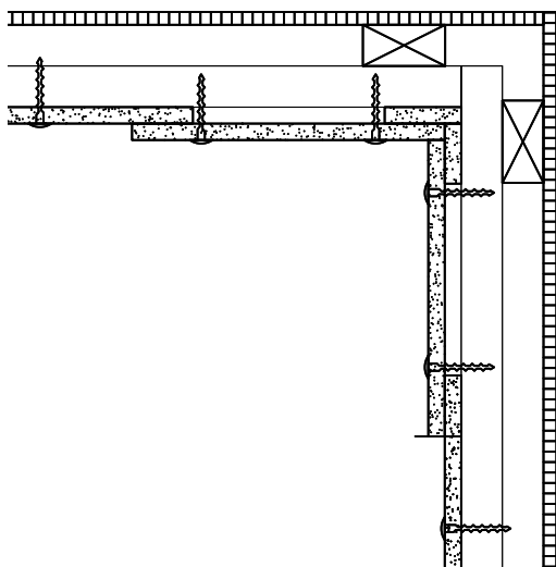
Konstruktionsprincip 2 uden profiler.
