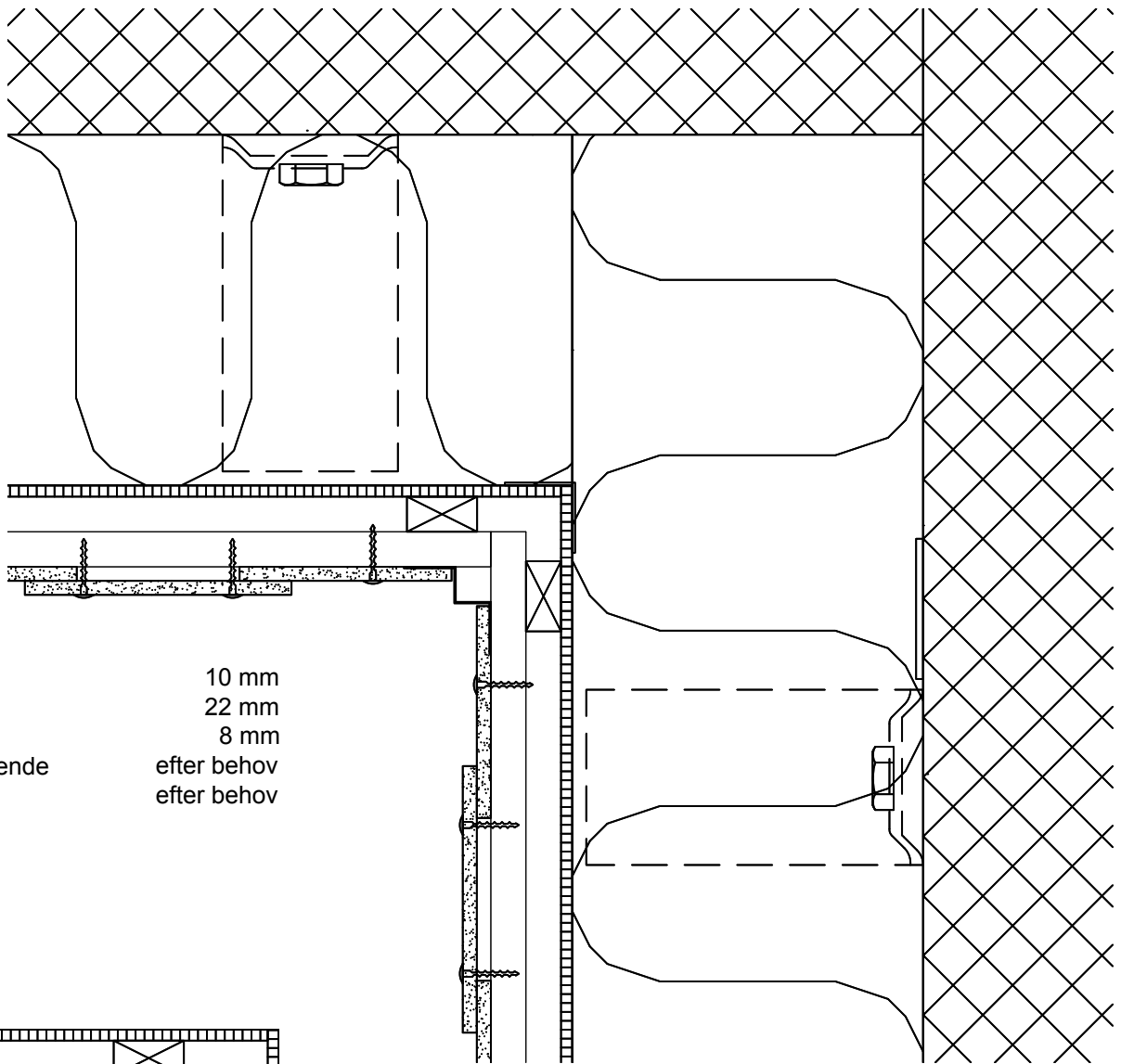
Konstruktionsprincip 1 med hjørneprofil.
