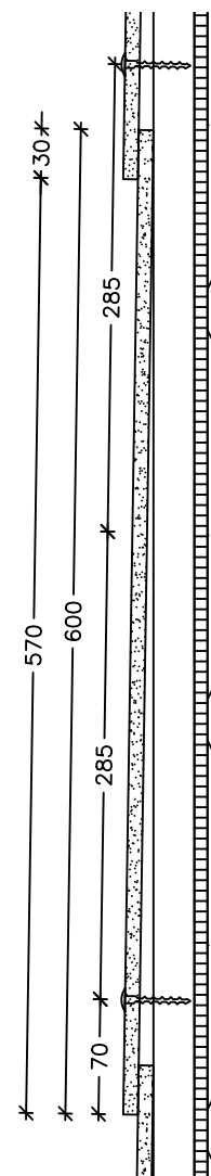
Lodret snit 1:5
