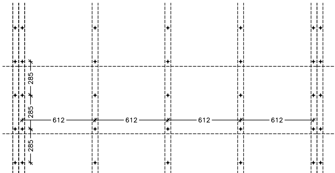
Opstalt af en hel plade 1:20
