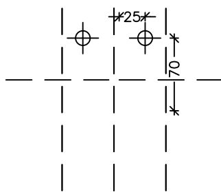
Opstalt ved lodret og vandret samling 1:5
